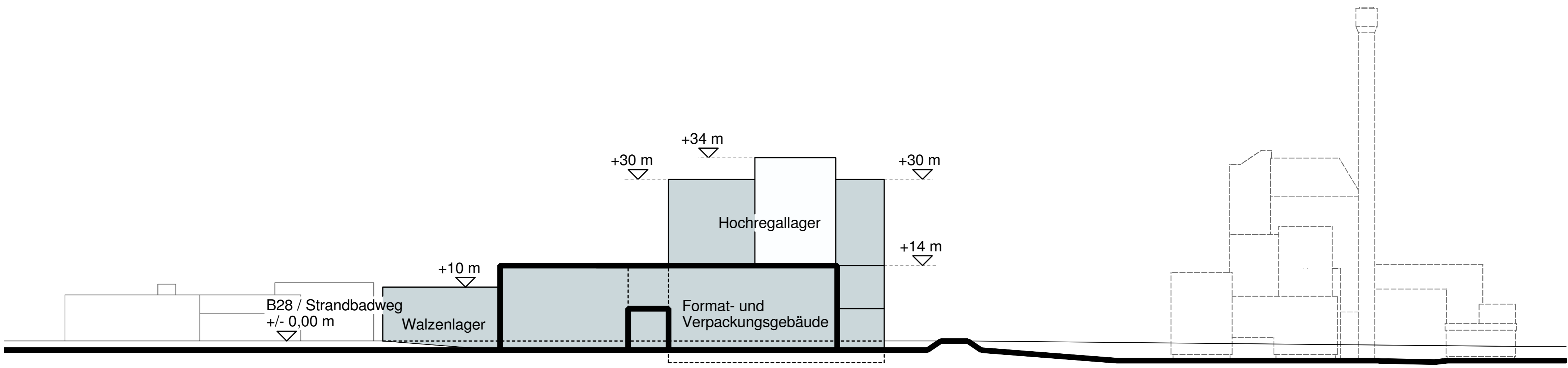
ANSICHT VON WESTEN
